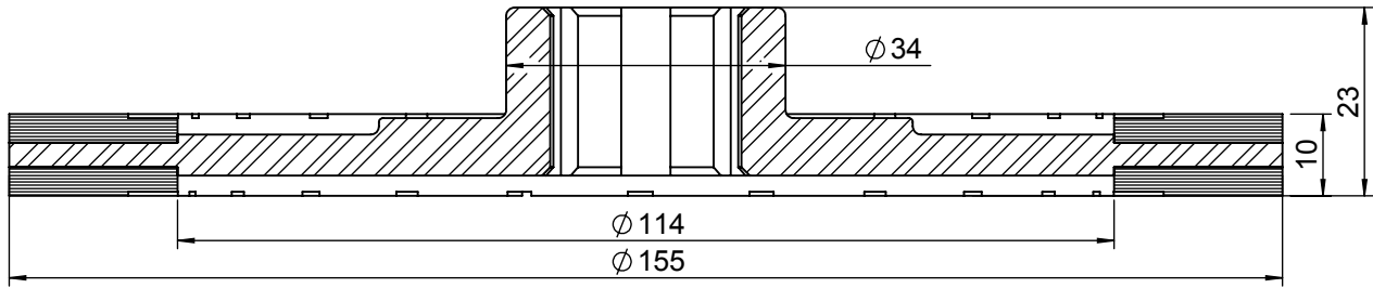
SEZIONE A-A
