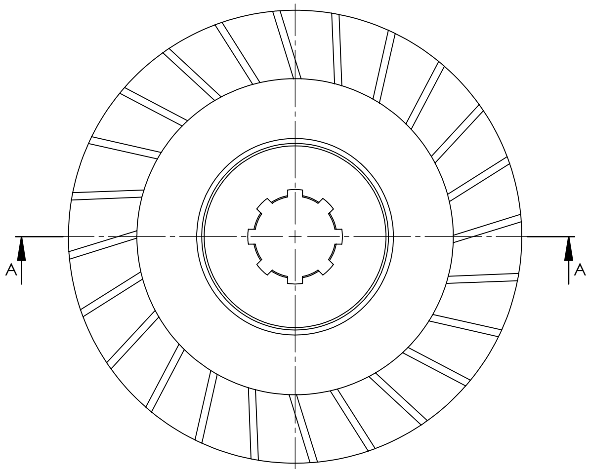
SEZIONE A-A
