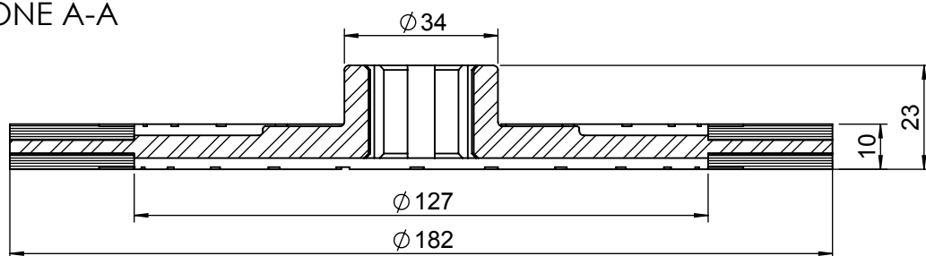
SEZIONE A-A
