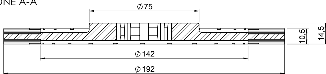
SEZIONE A-A
