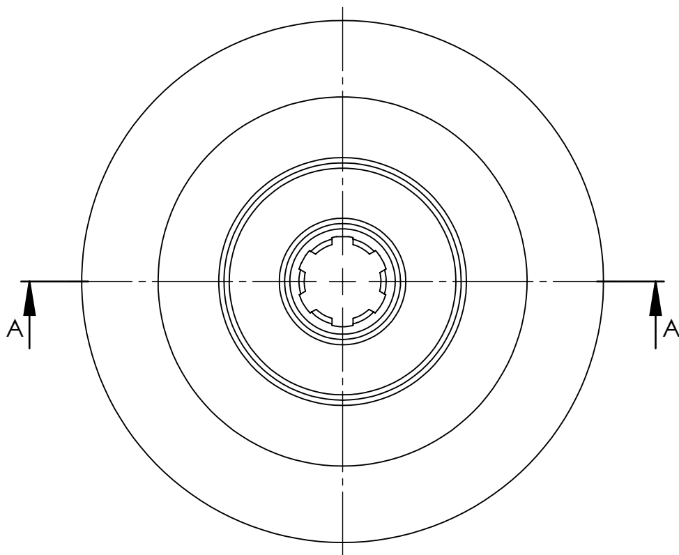
SEZIONE A-A
