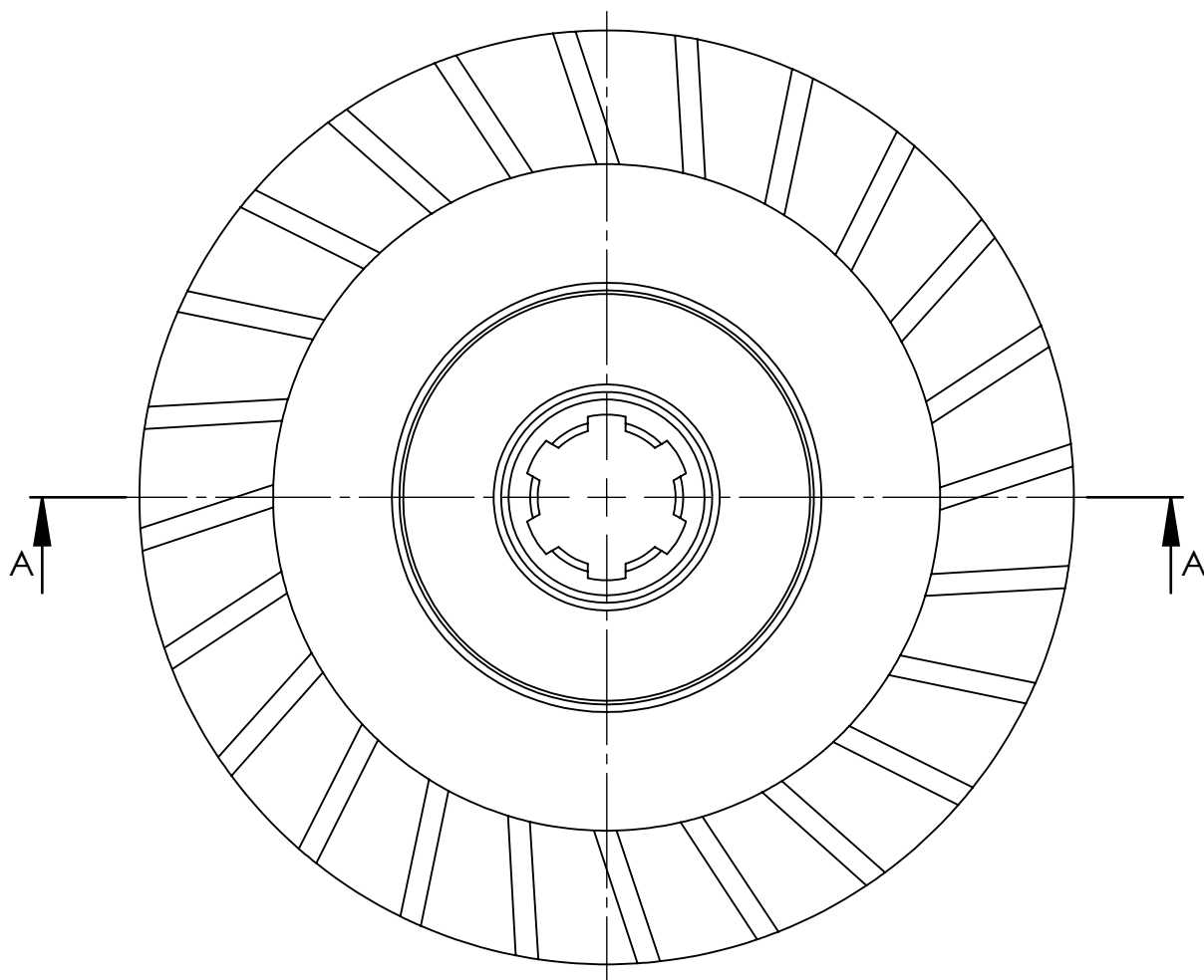
SEZIONE A-A
