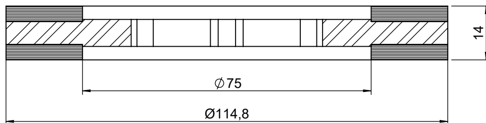
SEZIONE A-A
