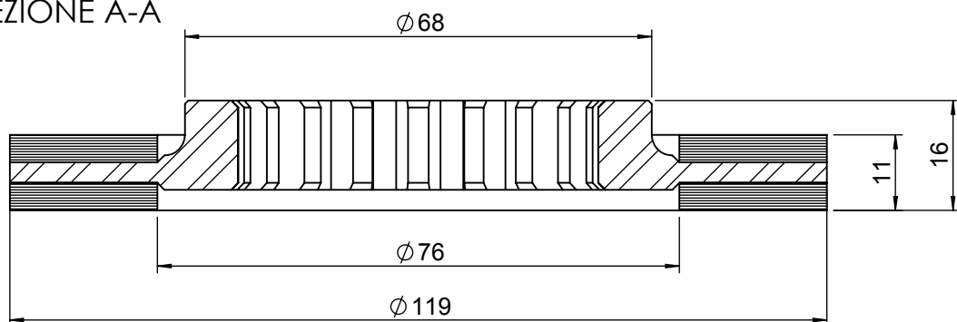
SEZIONE A-A
