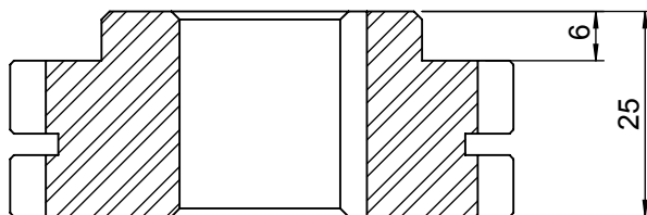
SEZIONE A-A
