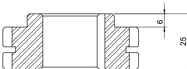
SEZIONE A-A
