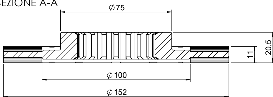
SEZIONE A-A
