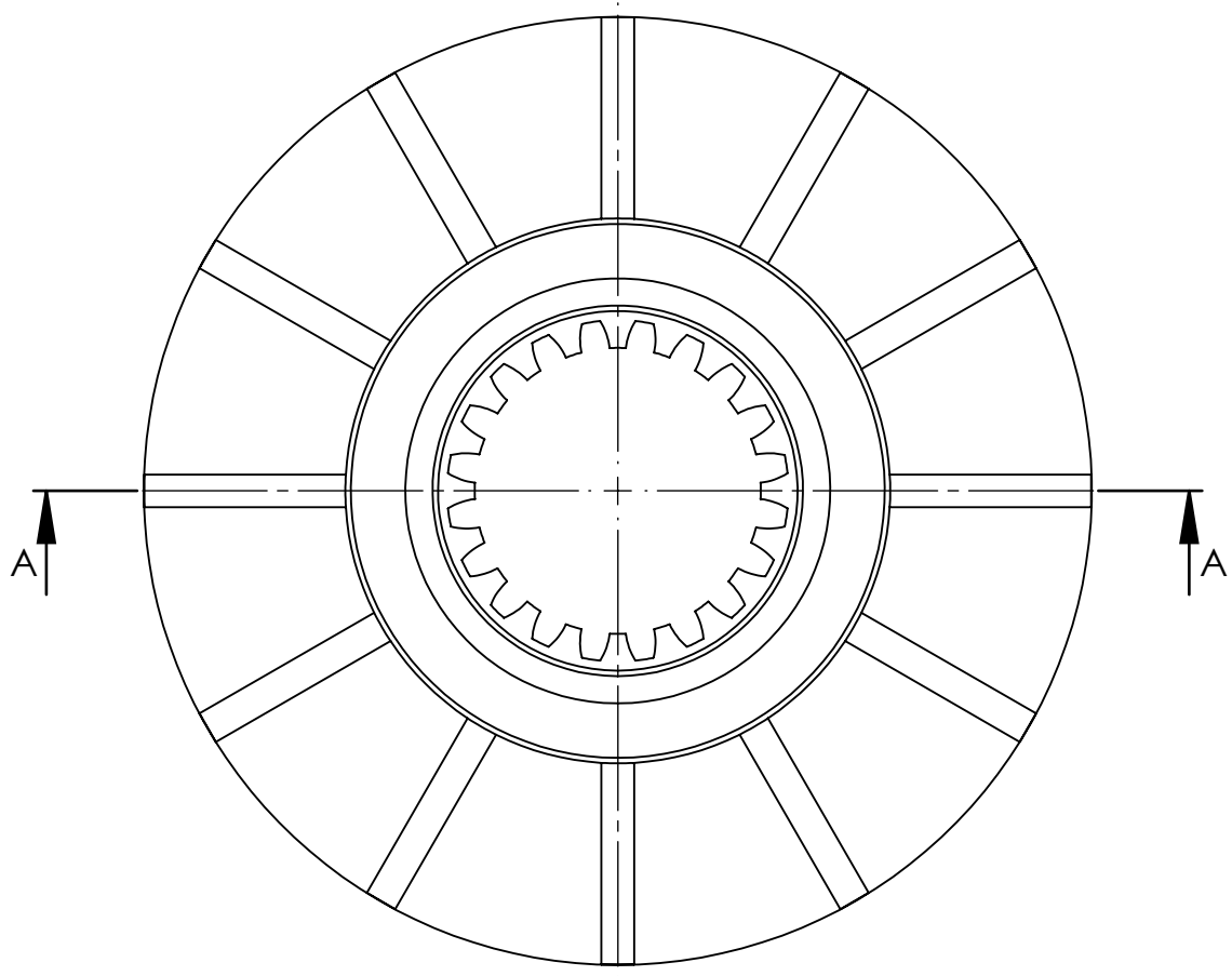
SEZIONE A-A
