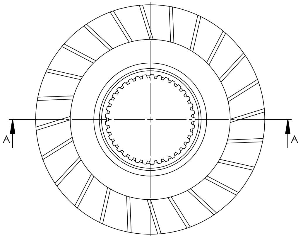
SEZIONE A-A
