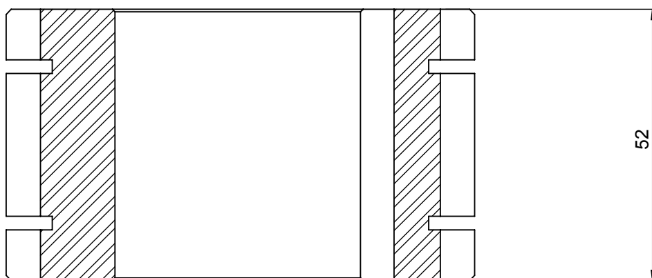
SEZIONE A-A
