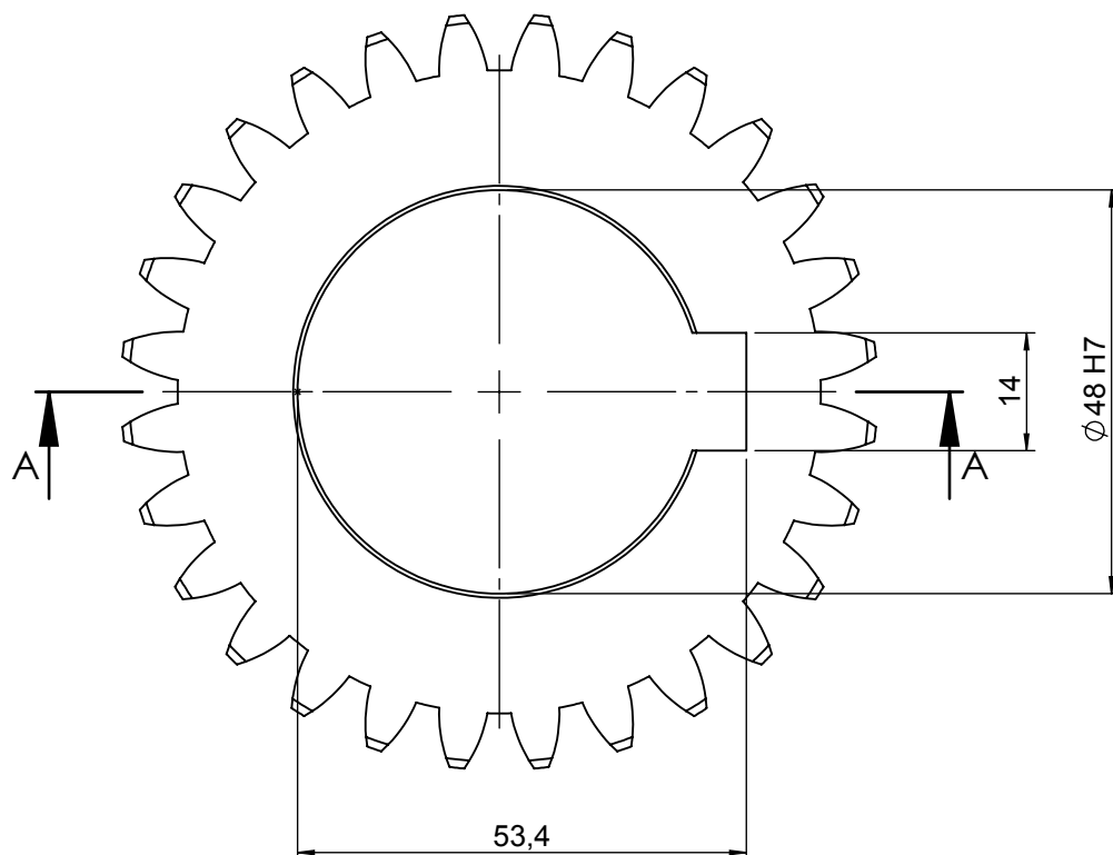
SEZIONE A-A
