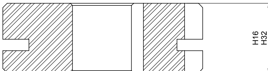
SEZIONE A-A
