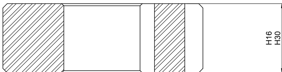
SEZIONE A-A
