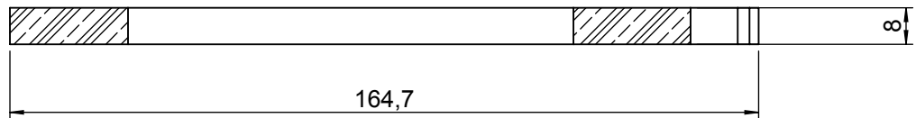
SEZIONE A-A
