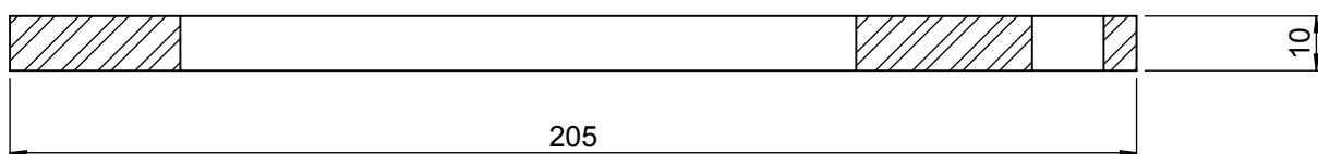
SEZIONE A-A
