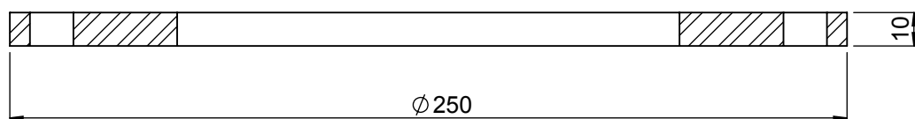
SEZIONE A-A
