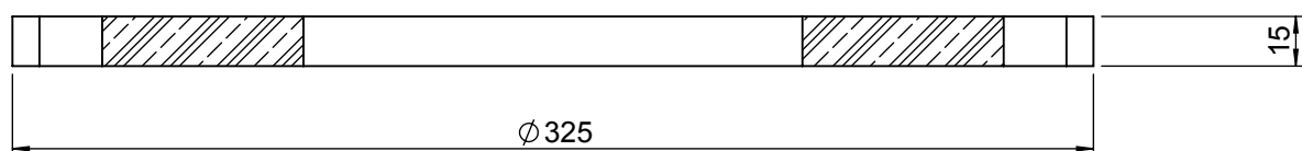
SEZIONE A-A
