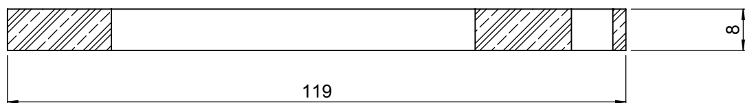
SEZIONE A-A
