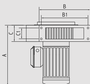
VISTA LATERALE
